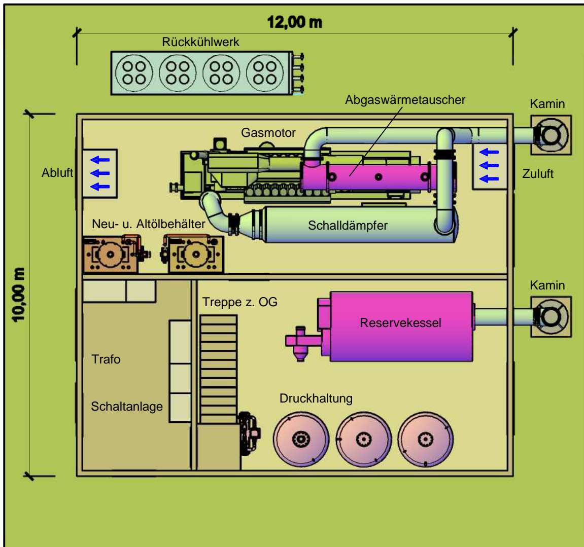
Grundriß EG
