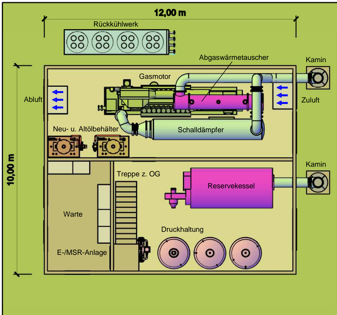
Grundriß OG
